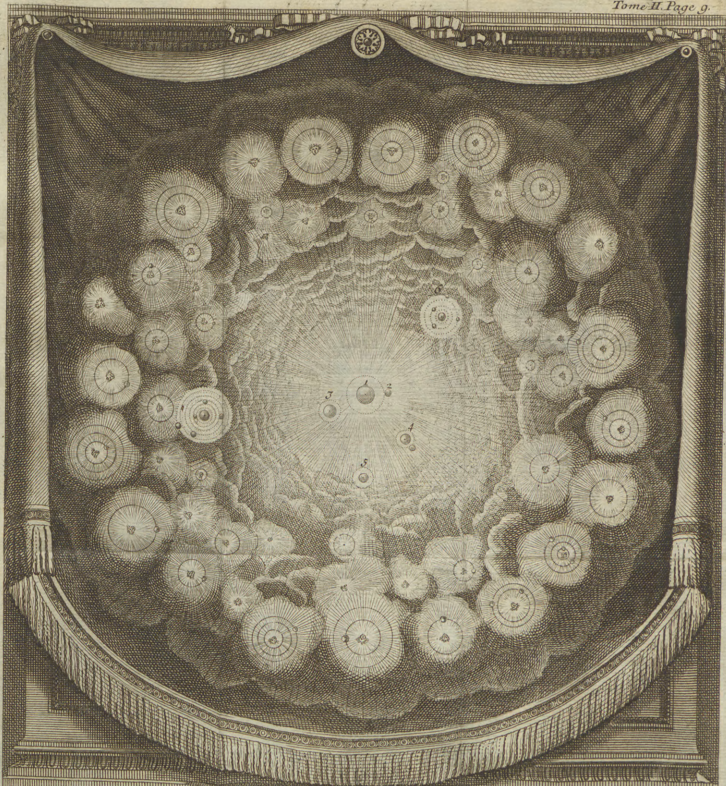
1 Le Soleil. 2 Mercure. 3 Venus. 4 La Terre. 5 Mars. 6 Jupiter. 7 Saturne.
